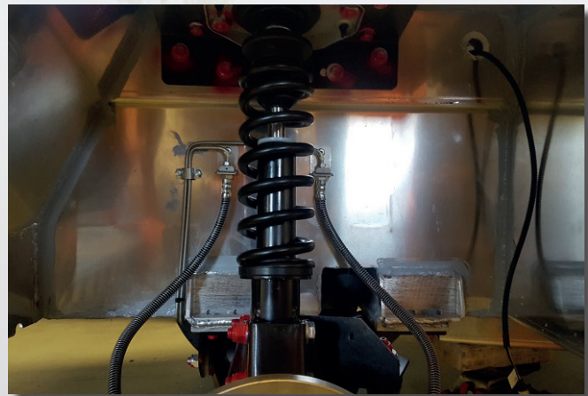
Hydraulisk stötdämpare med fjäder
