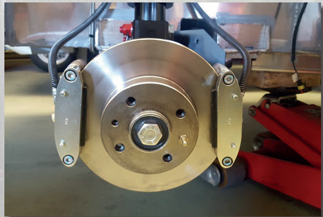
2 krets bromssystem med 4 bromsok för bättre säkerhet
